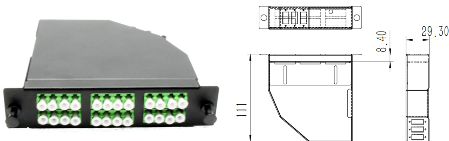
3xMPO/MTP-LC DX 8F
